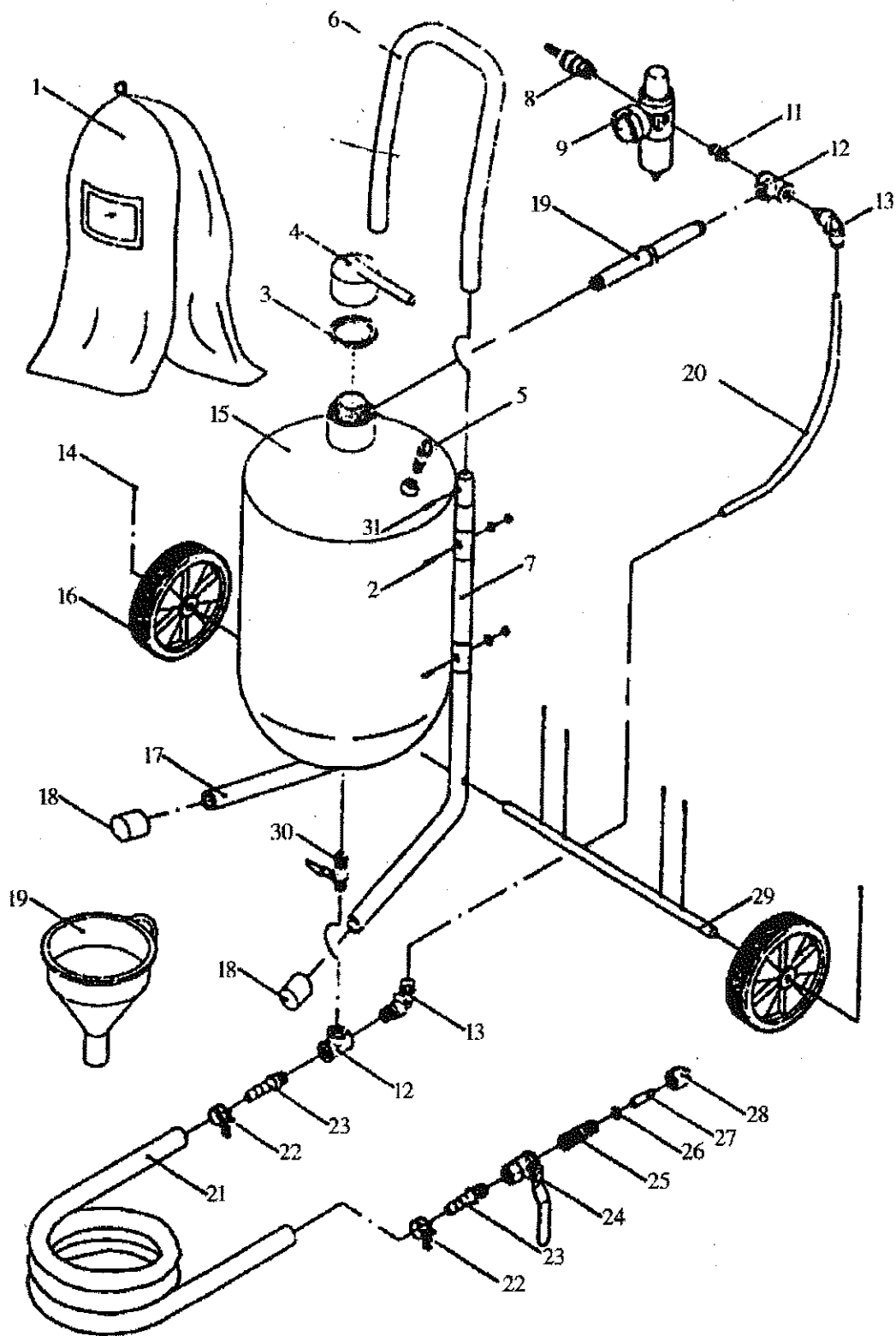
KUVA HIEKKAPUHALTIMEN OSISTA
