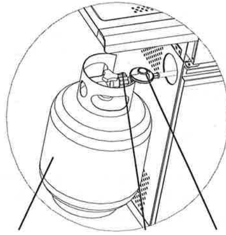
Kaasupullo Paineensäädin Letku Kaasupullon, paineensäätimen ja letkun liittäminen
